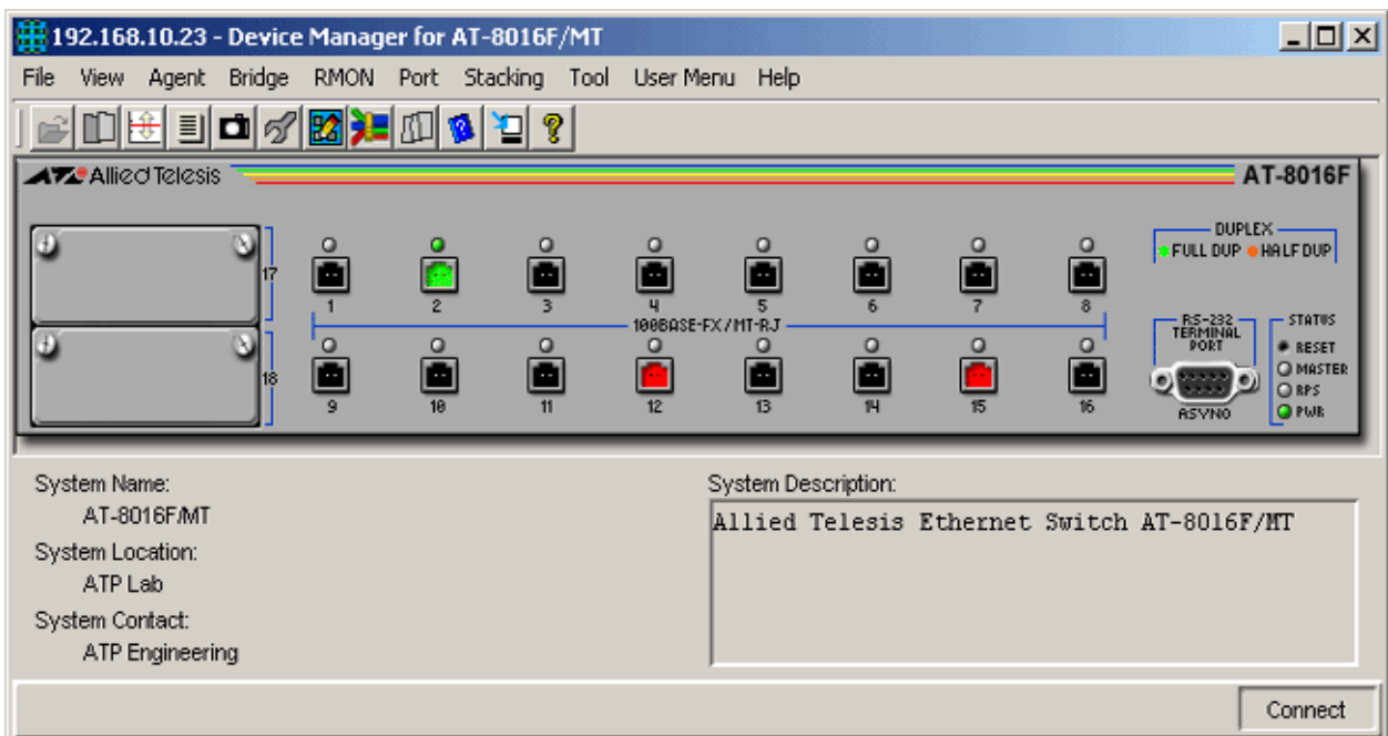
AT-8016F/MT
