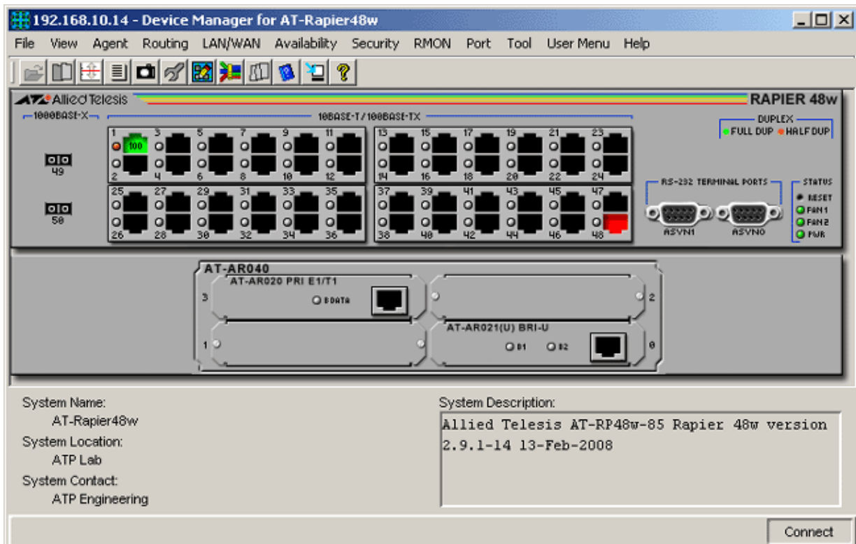
AT-Rapier 48w
